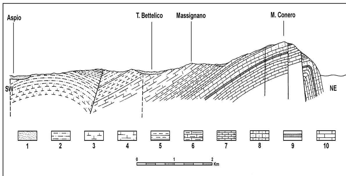
Fig. 4.1 – Sezione geologica dell'area del Conero: 1-Alluvioni 2-Marne a sabbie 3-Marne a colombacci 4-Schlier 5-Bisciaro 6-Scaglia cinerea 7-Scaglia Rosata 8-Scaglia Bianca 9-Marne a furoidi 10-Maiolica (da Cello e Coppola, 1983 – ridisegnato ) del Pliocene inferiore e medio e del Pleistocene con i litotipi marnoso-arenacei e argillosi.
