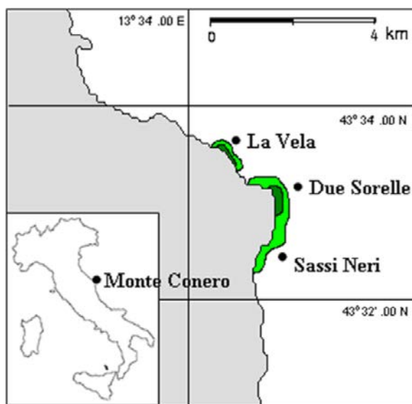
➤ Figura 1: Cambiamento nella distribuzione di canopy a Cystoseira tra il 2001 (verde chiaro) e il 2006 (verde scuro), da Petrol-Finkel & Airoidi 2010
